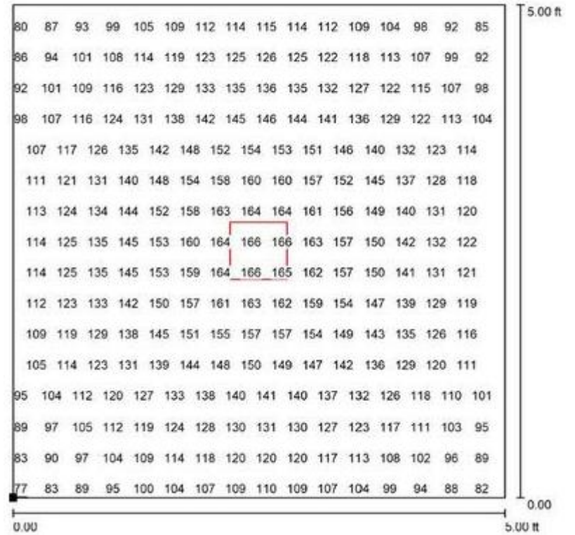
602 PAR Map - 5ft
